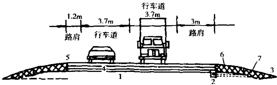
附图 6.1.5-2 路面典型横断面
