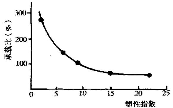
附图 6.2.5 塑性指数对级配集料承载比的影响
