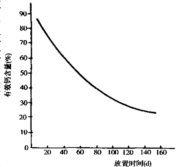
附图 4.2.2 放置时间对石灰有效钙含量的影响
