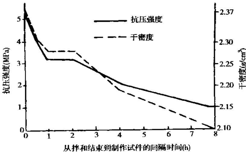
附图 3.1.7 延迟时间对水泥砂砾的强度和干密度的影响
