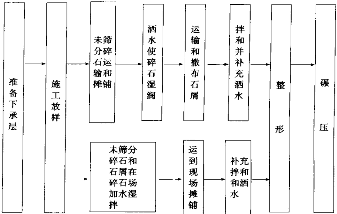
图 6.3.1 级配碎石路拌法施工工艺流程图
