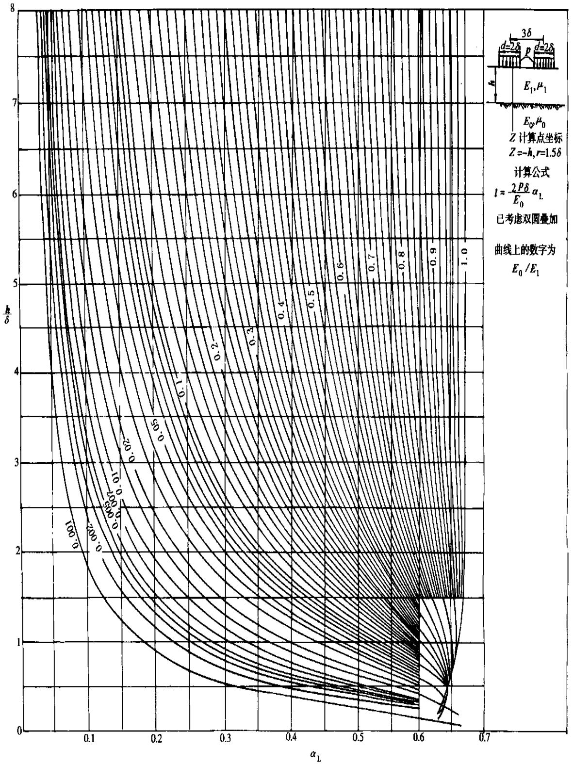
附图 A.0.3 双层体系表面弯沉系数图
