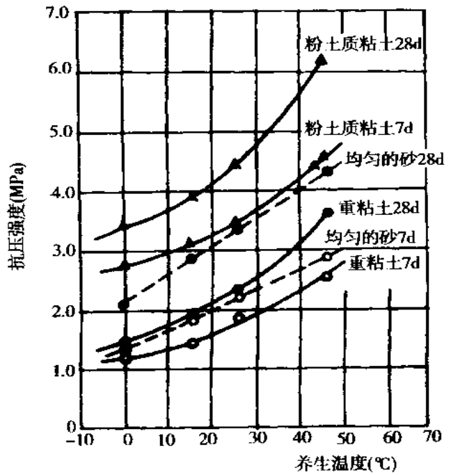
附图 3.1.5 养生温度对水泥稳定土抗压强度的影响
