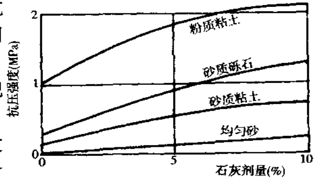
附图 4.2.1 土质对石灰稳定土抗压强度的影响
