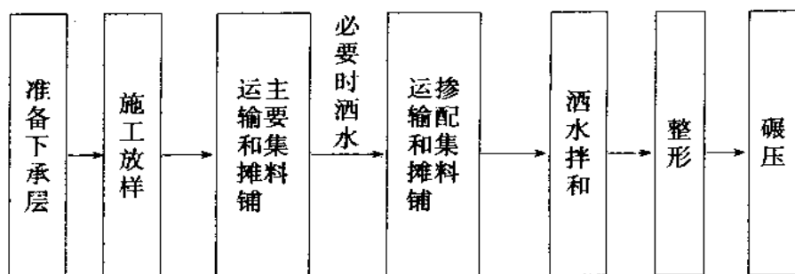
图 7.3.1 级配砾石施工工艺流程图
