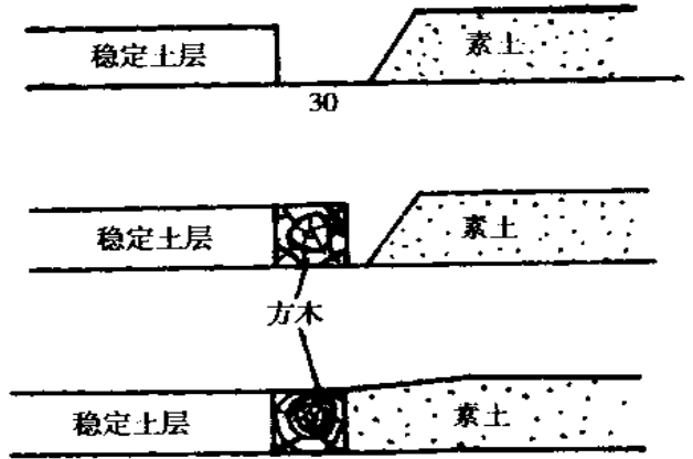
图 3.4.13 横向接缝处理示意图
