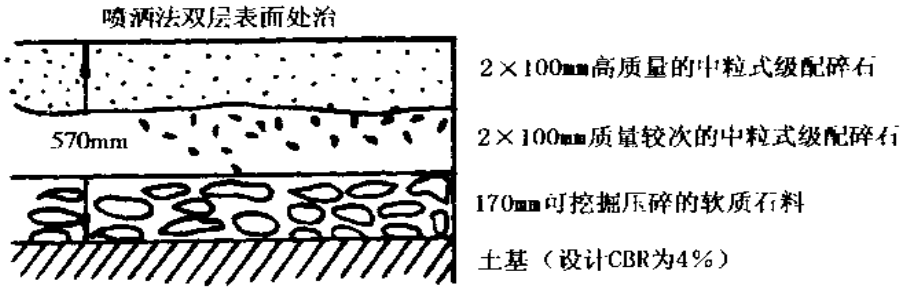
附图 6.1.5-1 维多利亚州重负荷柔性路面的典型结构
