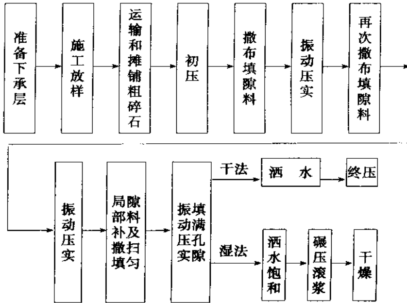
图 8.3.1 填隙碎石工艺流程图
