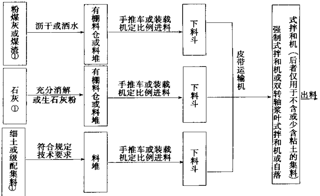
图 5.5.2 石灰工业废渣稳定土的集中拌和工艺流程②
