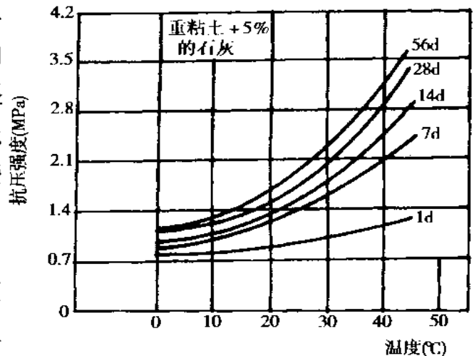
附图 4.1.5 养生温度对石灰稳定土抗压强度的影响
