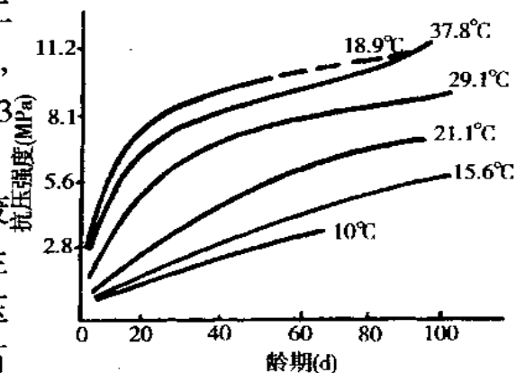
附图 5.1.5 养生温度对二灰砂砾抗压强度的影响
