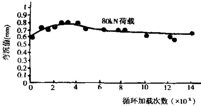
附图 6.1.5-3 级配碎石沥青表面 处治弯沉演变图
