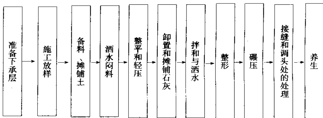
图 4.4.1 石灰稳定土路拌法施工的工艺流程
