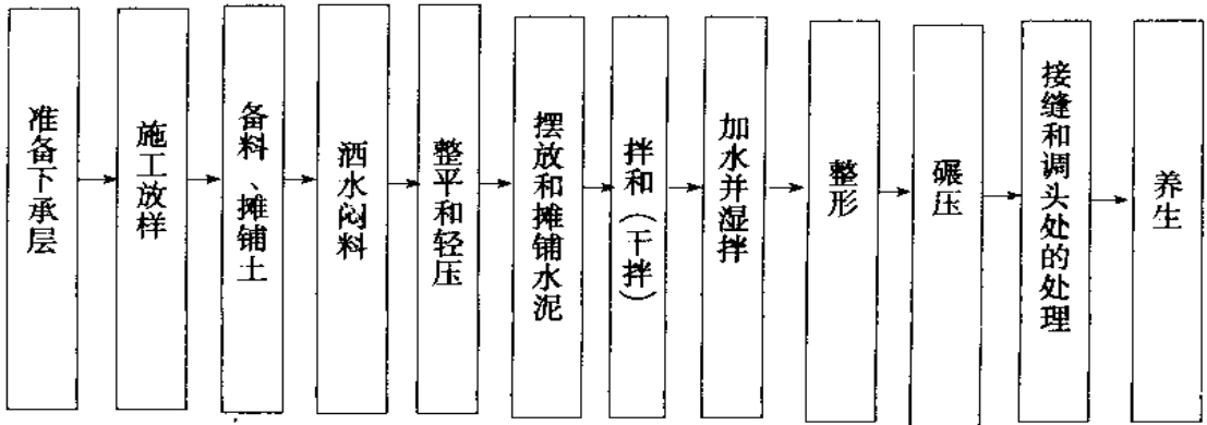
图 3.4.1 路拌法施工水泥稳定土的工艺流程
