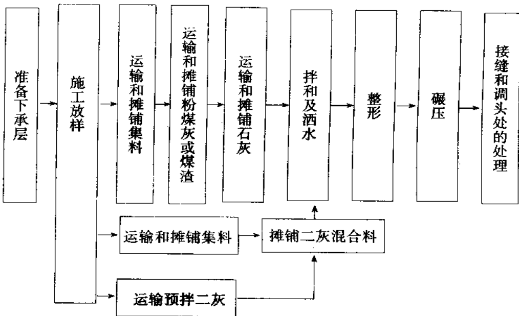
图 5.4.1 路拌法施工石灰工业废渣稳定土的工艺流程图
