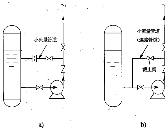
图 C.2-2 小流量管道
