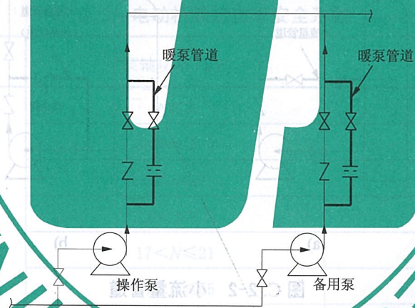
图 C. 2-5 暖泵管道（冷泵管道）
