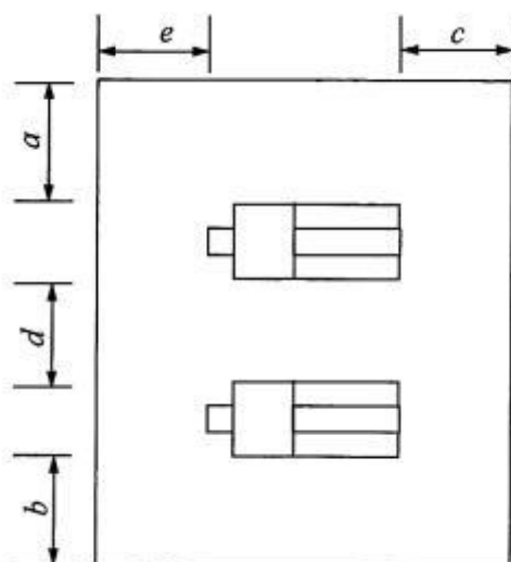
图 6.1.4 机组布置
