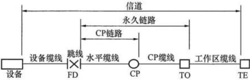
图 21. 2. 5-1 配线子系统线缆划分
