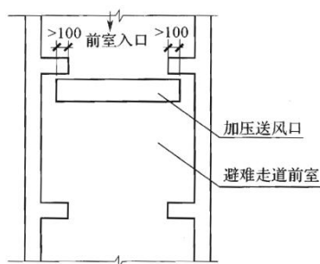
图 6.2.2 避难走道前室加压送风口布置图
