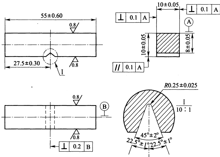
图 D. 2. 3-1 V 形缺口冲击试样
