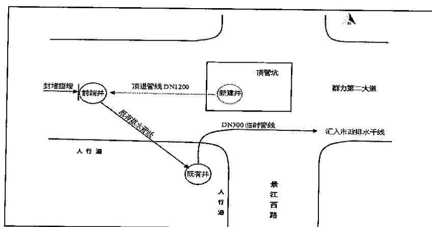
工程平面示意图
