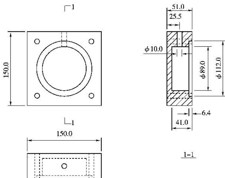
图 A.2.2 试验槽结构图(mm)
