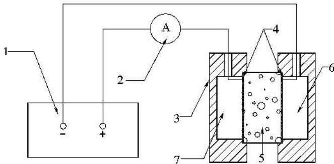
图 A.2.1 试验装置示意图
