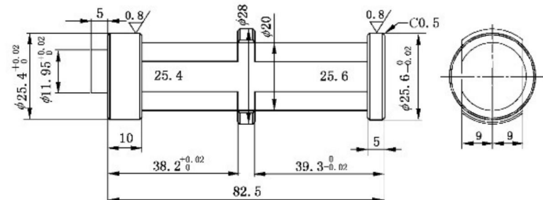
DC+/DC- 通止规 25.4
