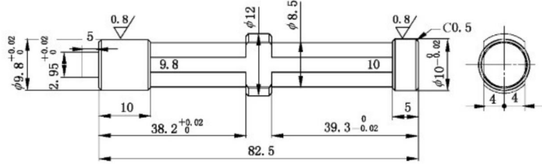
CC2 通止规 9.8
