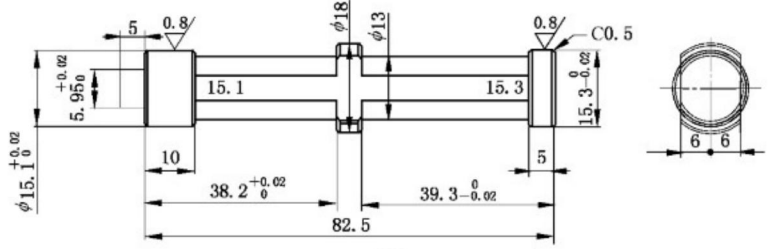
PE 通止规 15.1
