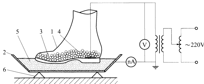
1—被试靴；2—金属盘；3—金属球；4—金属片；5—海绵和水；6—绝缘支架
