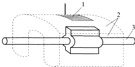
图 B.3 绝缘罩试验电极布置示意图
