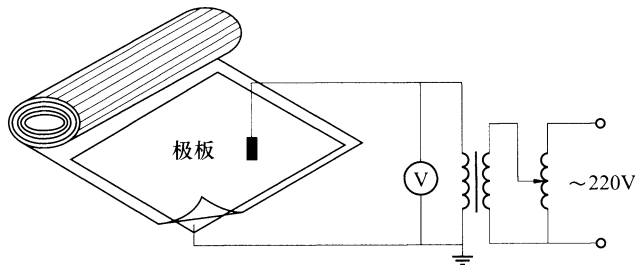
图 B.6 辅助型绝缘胶垫试验接线图
