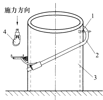
1—限位装置；2—登杆脚扣；3—模拟电杆；4—鞋模
