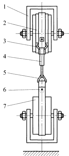
1—夹具；2—安全带；3—半圆环；4—钩；5—三角环；6—带、绳；7—木轮
