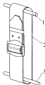
1—上夹具销轴；2—扣带；3—下夹具销轴
