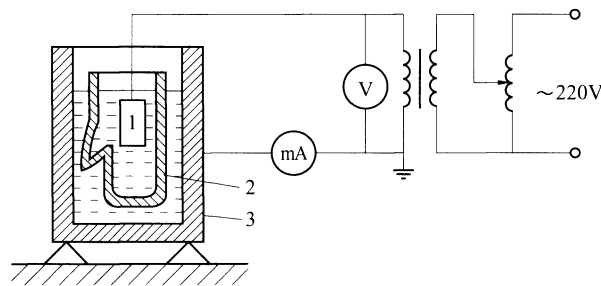
1—电极；2—试样；3—盛水金属器皿
