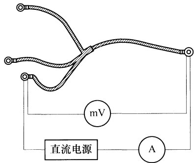
图 B.1 个人保安线、携带型短路接地线线鼻子间成组直流电阻试验接线图
