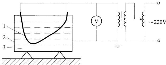
图 B.2 核相器连接导线绝缘强度试验接线图
