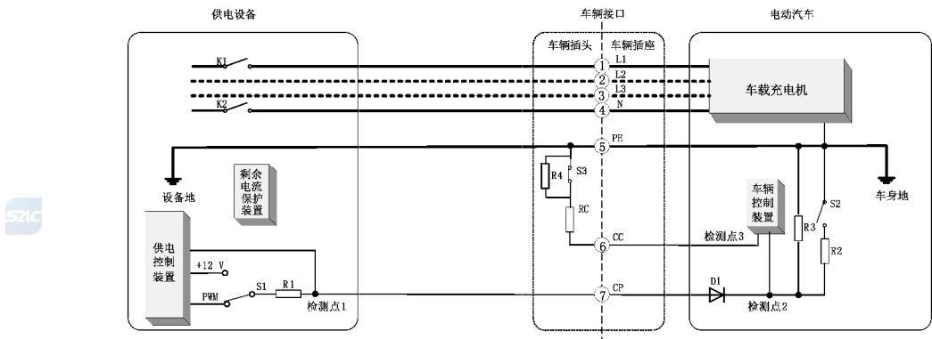
图 A.3 充电模式 3 连接方式 C 的控制导引电路原理图
