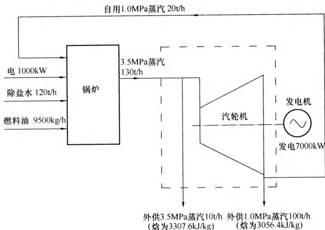
图1 动力站设计能源折算值计算示意图
