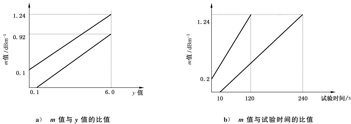
图 I.1 试验火合格判据
