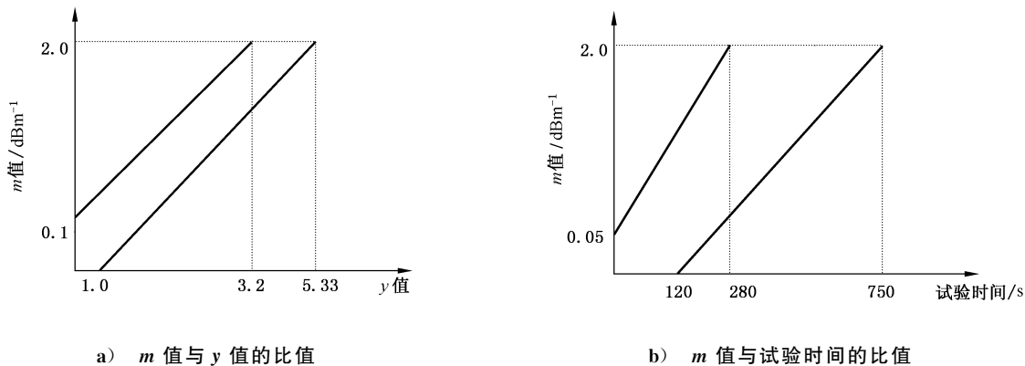
图 G.2 试验火合格判据
