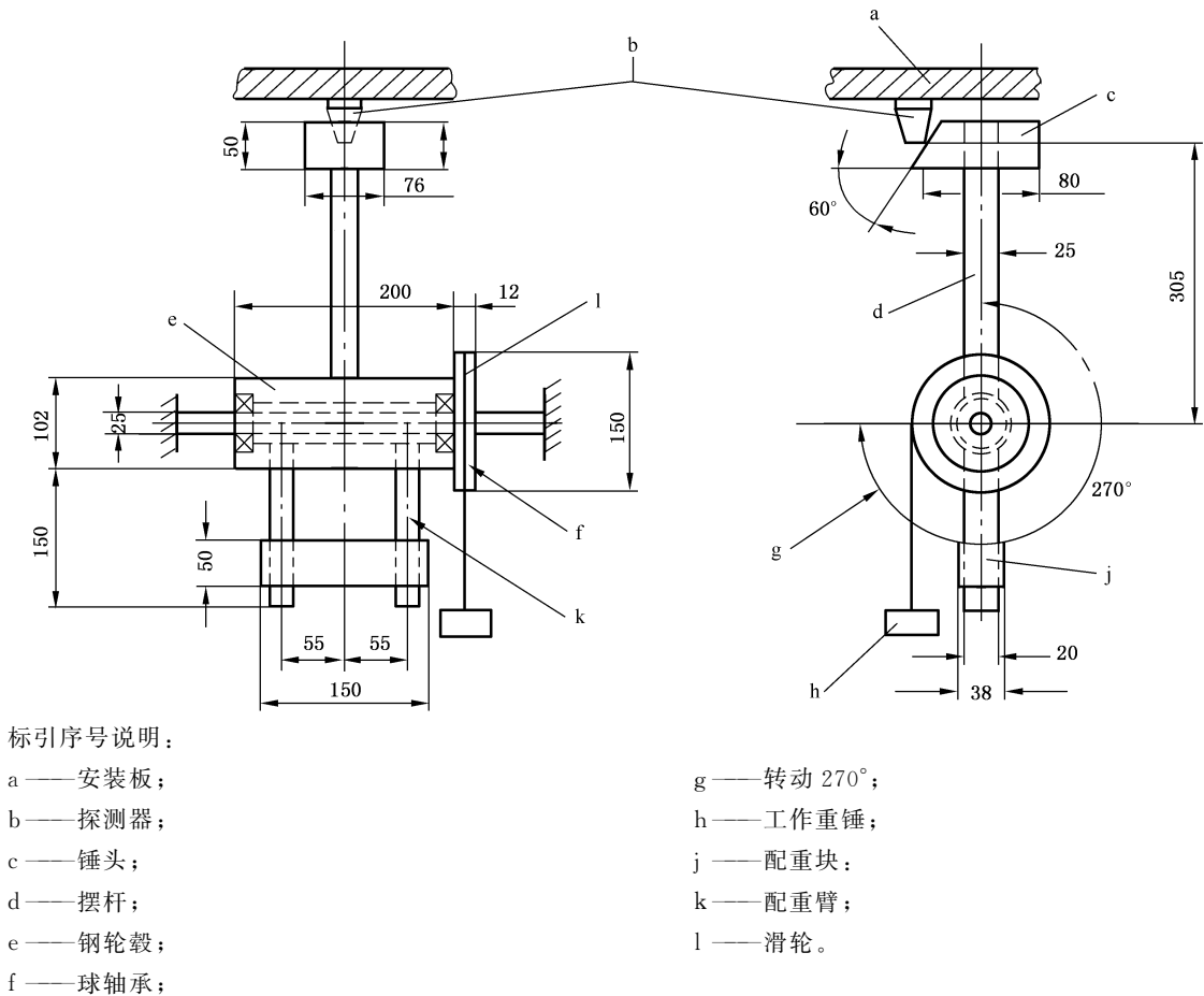
图 D.1 碰撞试验设备图
