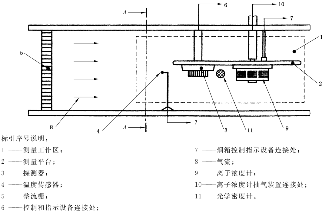
图 A.1 测量区、试验仪器及探测器的布置图(一)
