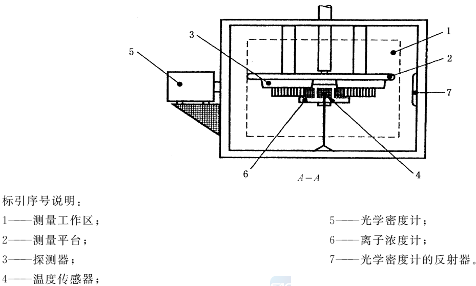
图 A.2 测量区、试验仪器及探测器的布置图(二)
