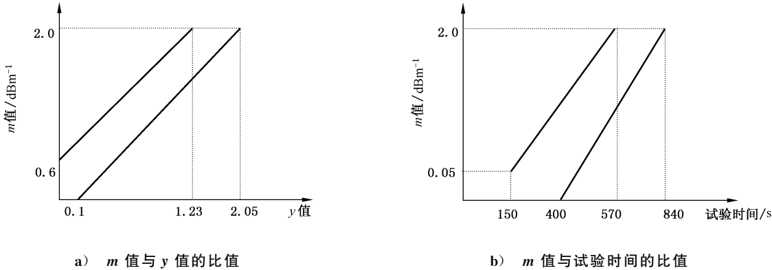
图 F.2 试验火合格判据
