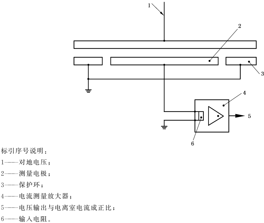
图 A.5 离子烟浓度计工作电路
