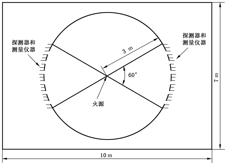
图 E.1 试验布置图
