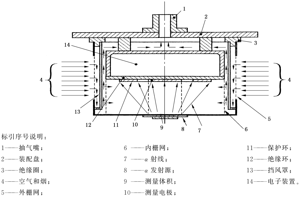
图 A.3 离子烟浓度计电离室工作原理
