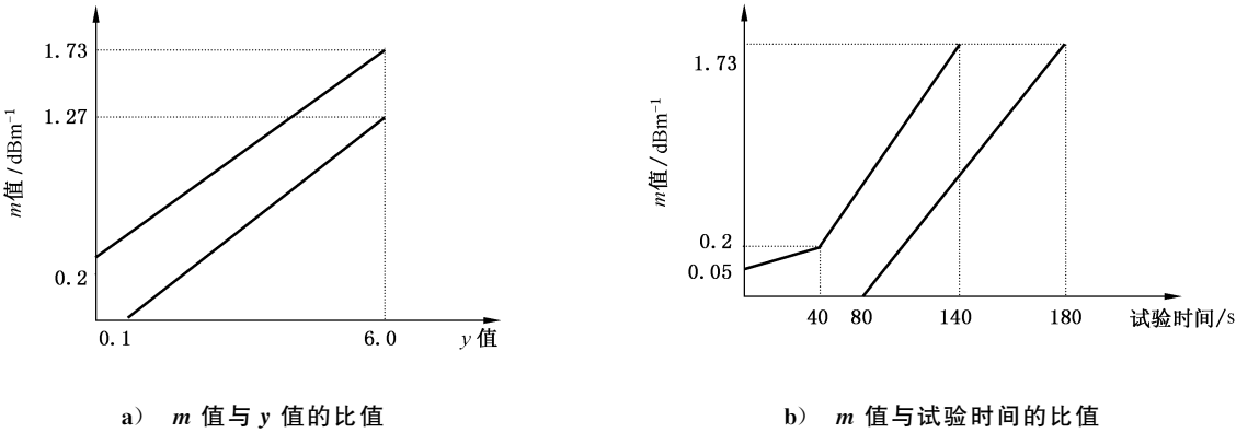
图 H.1 试验火合格判据
