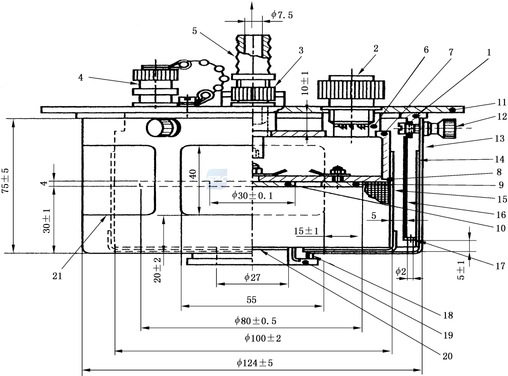
图 A.4 电离室结构图
