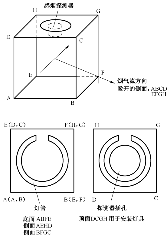
图 C.1 闪光装置图
