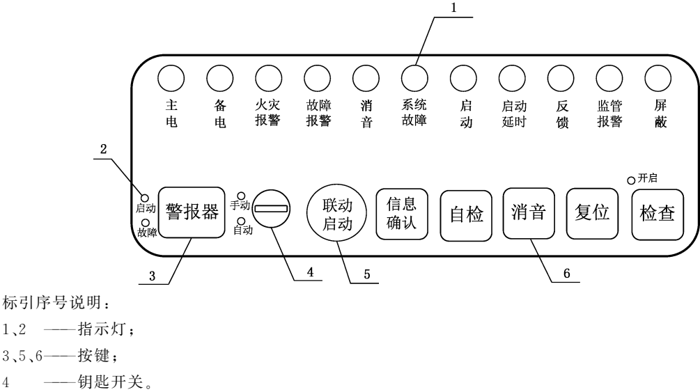
图 1 按键与指示灯横向设置
