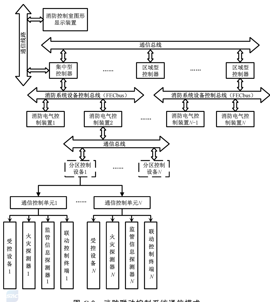
图 C.2 消防联动控制系统通信模式
