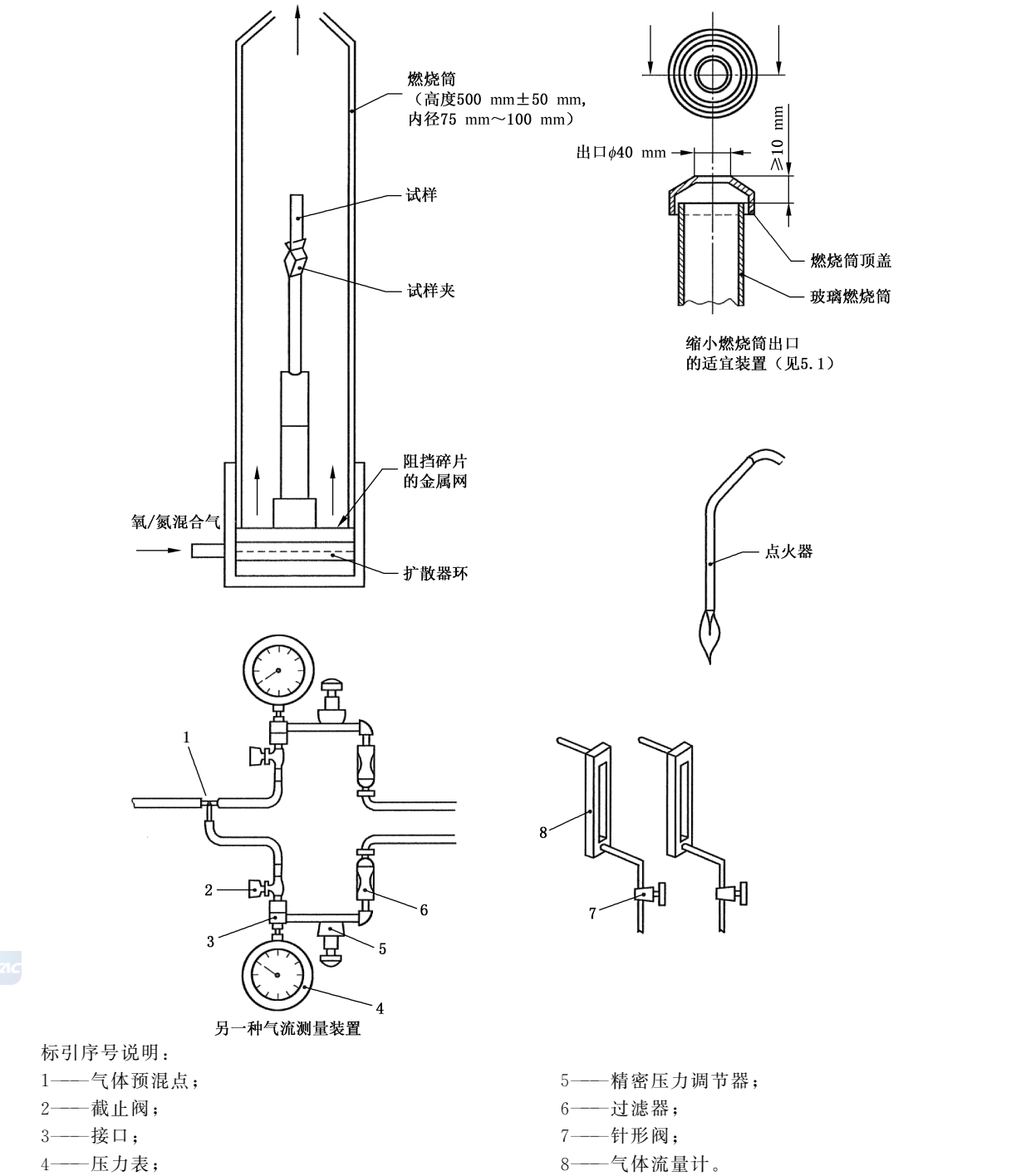
图 A.1 外壳燃烧性能试验设备
