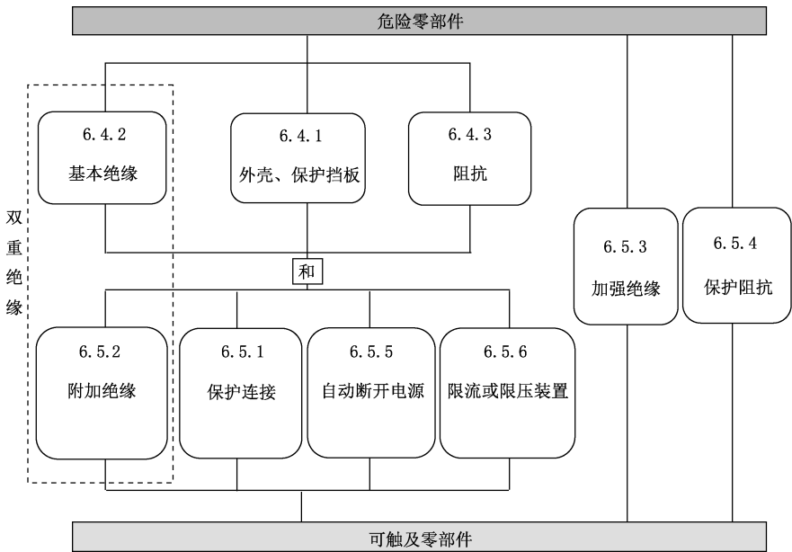
图 1 电击防护措施可接受的方案
